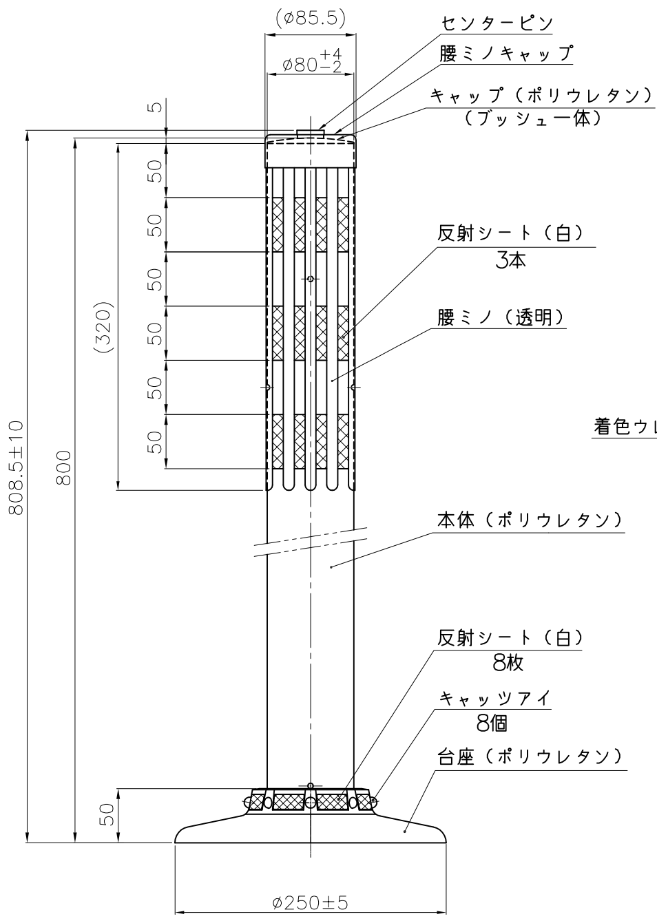
本体反射シート部詳細図
