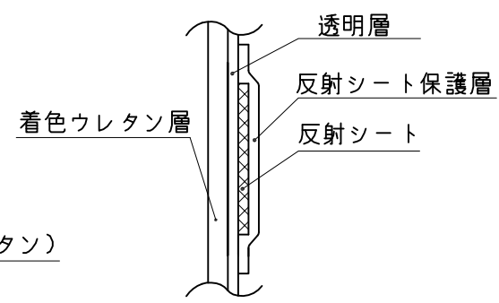
本体反射シート部詳細図
